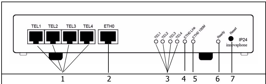
Abbildung 1 - Anzeigen und Anschlüsse der IP24
