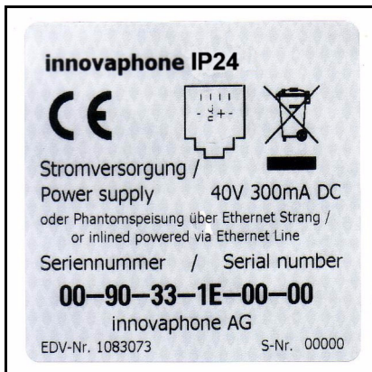
Abbildung 3 Das Seriennummernetikett der IP24
