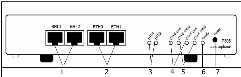
Abbildung 1 Anzeigen und Anschlüsse der IP305
